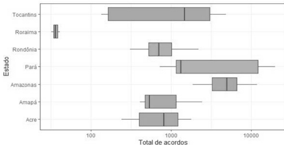
Figura 20 – Boxplot em escala logarítmica do número de acordos extrajudiciais dos Estados da região Norte do Brasil
