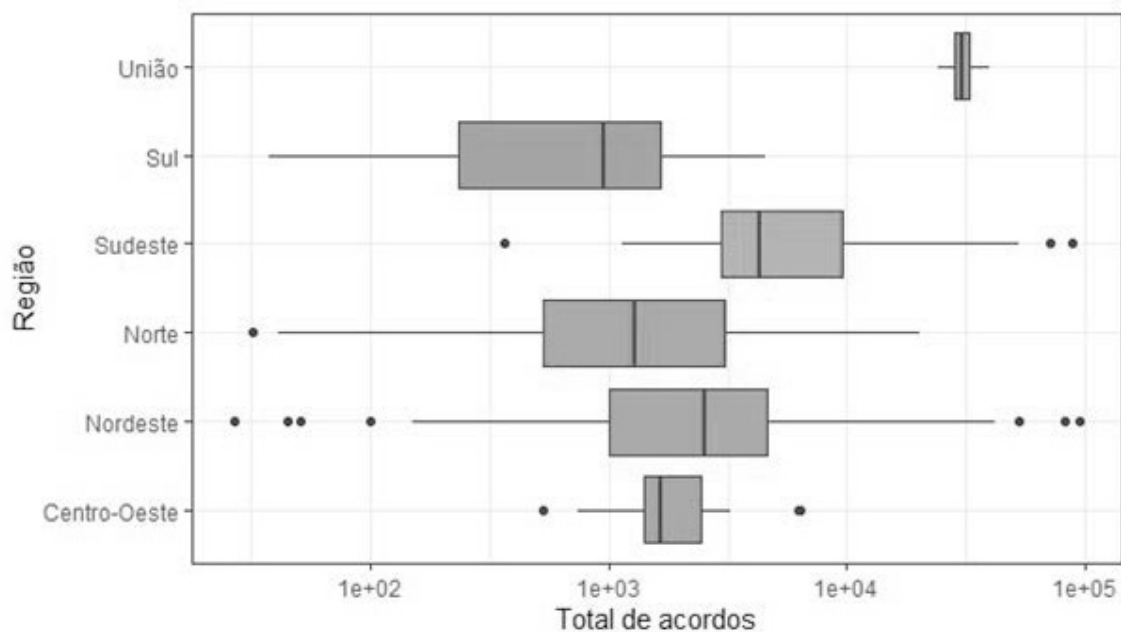
Figura 21 – Boxplot em escala logarítmica do número de acordos extrajudiciais das regiões do Brasil
